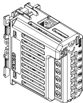
DESCRIZIONE MORSETTI
