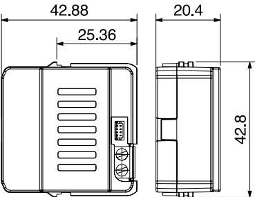
GW A1 700 Unità di alimentazione e connessione
