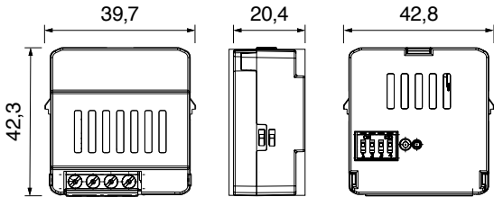
GW A1 521 Attuatore carichi generici 1 canale GW A1 523 Attuatore carichi generici 1 canale con misura di potenza
