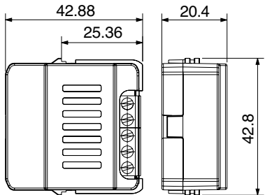
GW A1 918 Misuratore di energia connesso
