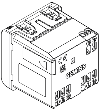
DESCRIZIONE MORSETTI
