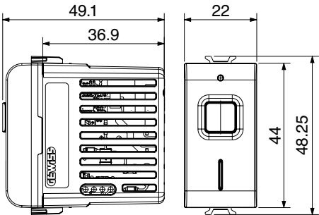
GW 1x 826 Attuatore connesso 1 canale con misura di energia
